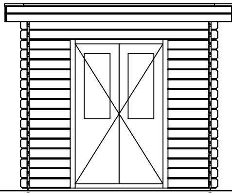
Voor-aanzicht / Front view / Vorderansicht
