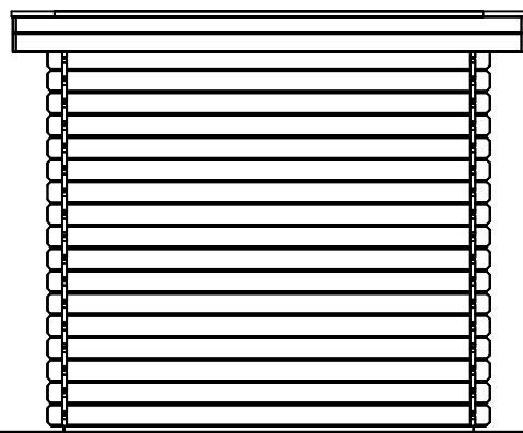
Achteraanzicht / Rear view / Hinterseite
