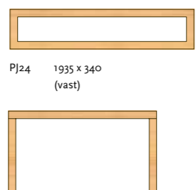
PJ05 340 x 730 (vast) PJ06 340 x 1140 (vast) PJ07 340 x 1530 (vast)
