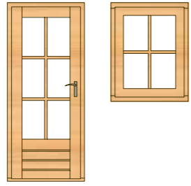
PX39 770 x 1800 PX39H 770 x 1935
