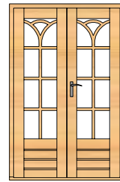
PE28 1210 x 1800 PE27 1210 x 1530 PE28H 1210 x 1935
