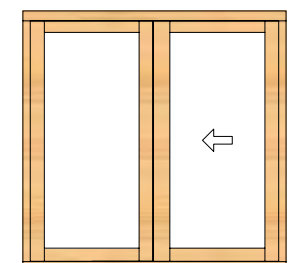
SD200 2000 x 1935 (schuif)
