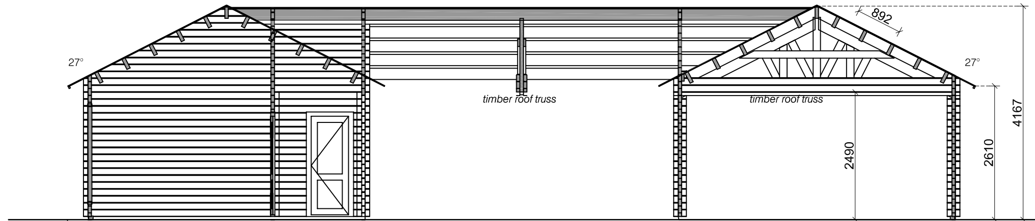
Doorsnede / Section / Durchschnitt A-A
