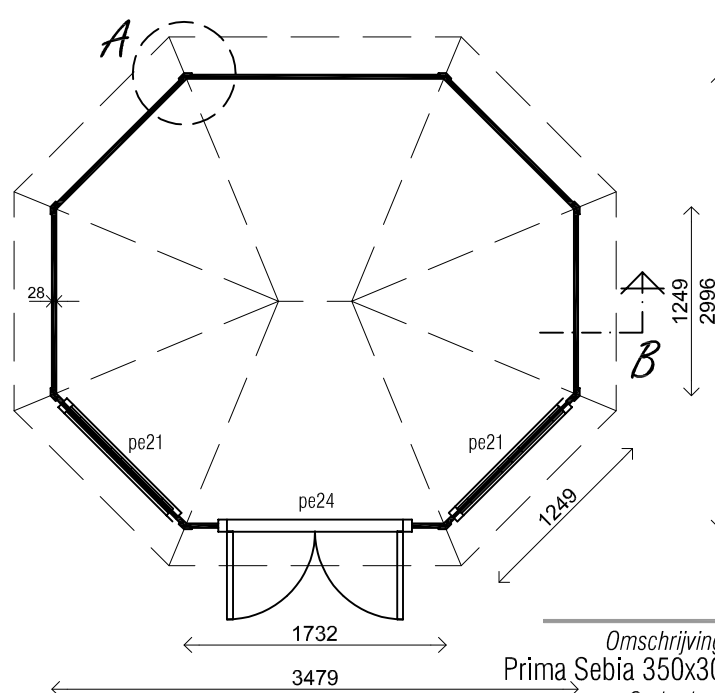
Plattegrond / Plan
